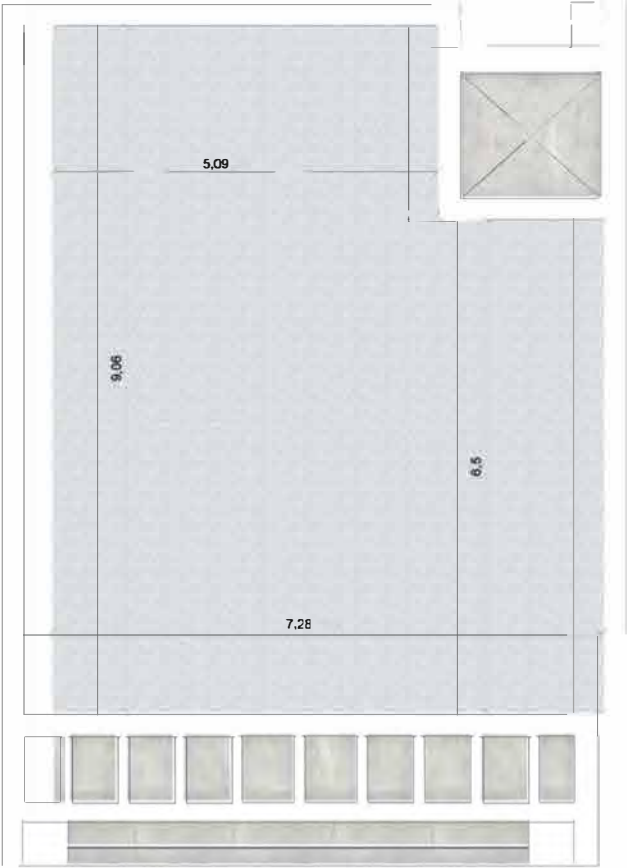
PLANTA DE CUBIERTA
