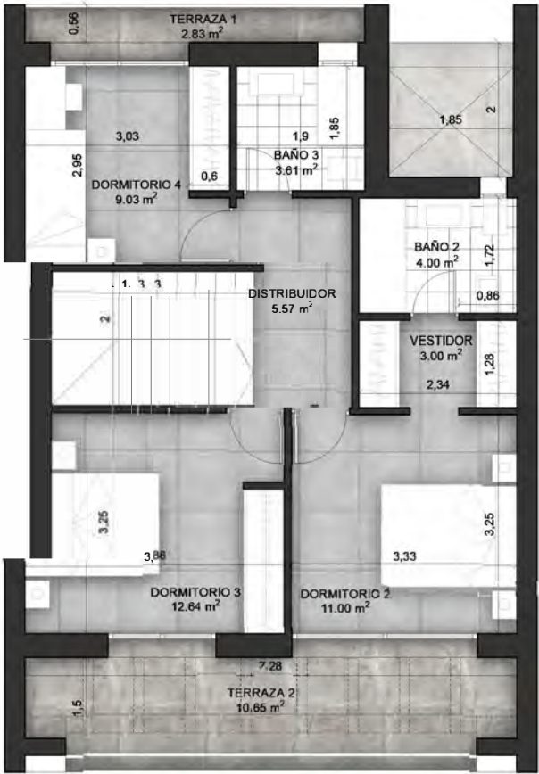
PLANTA PRIMERA
